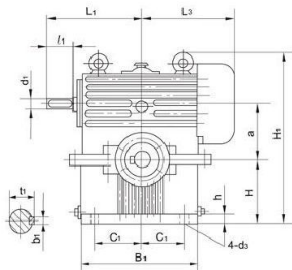
HWT型减速器外形尺寸及装配型式
