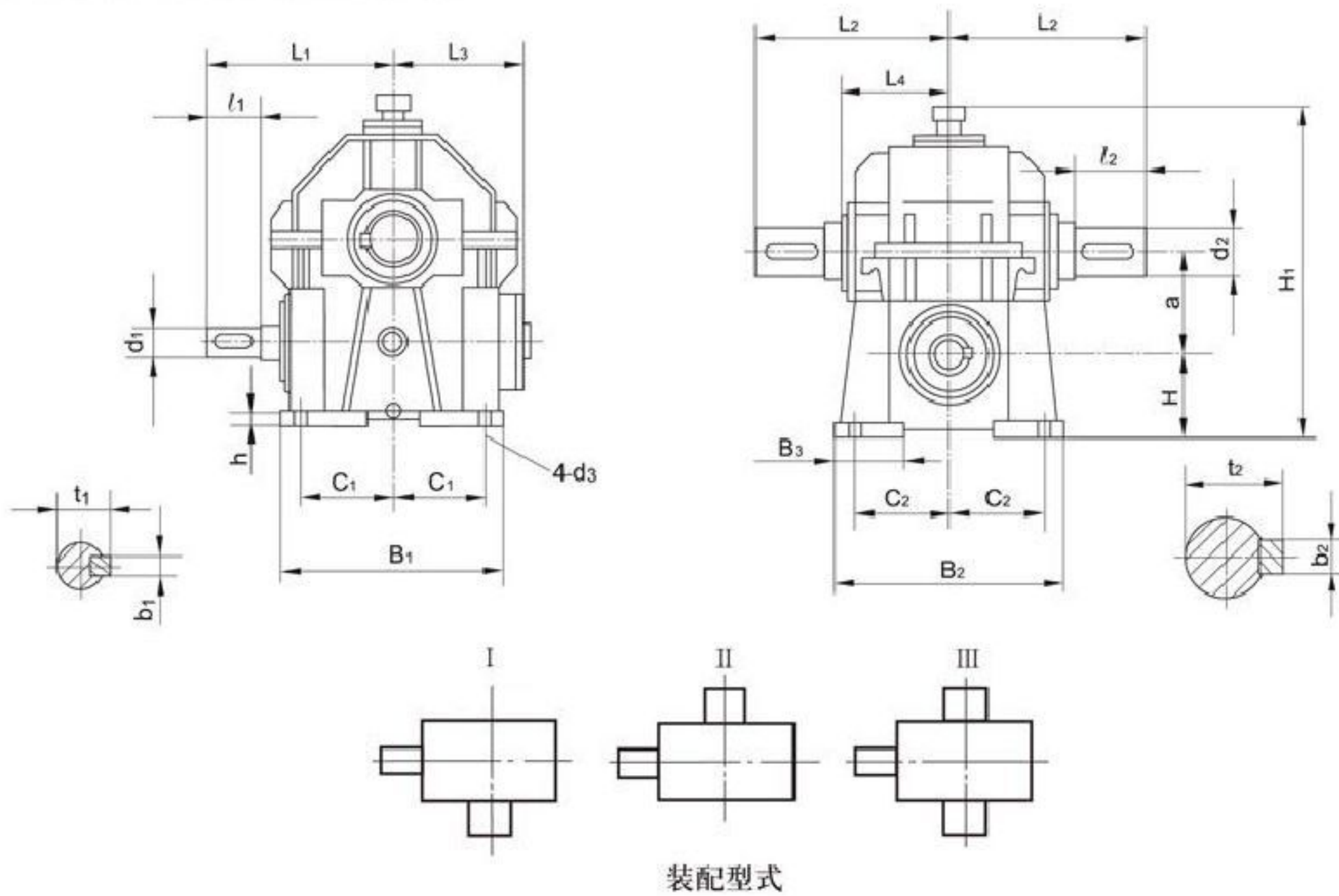
HWWB型减速器外形尺寸及装配型式
