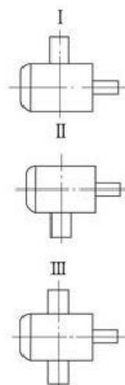
装配型式
