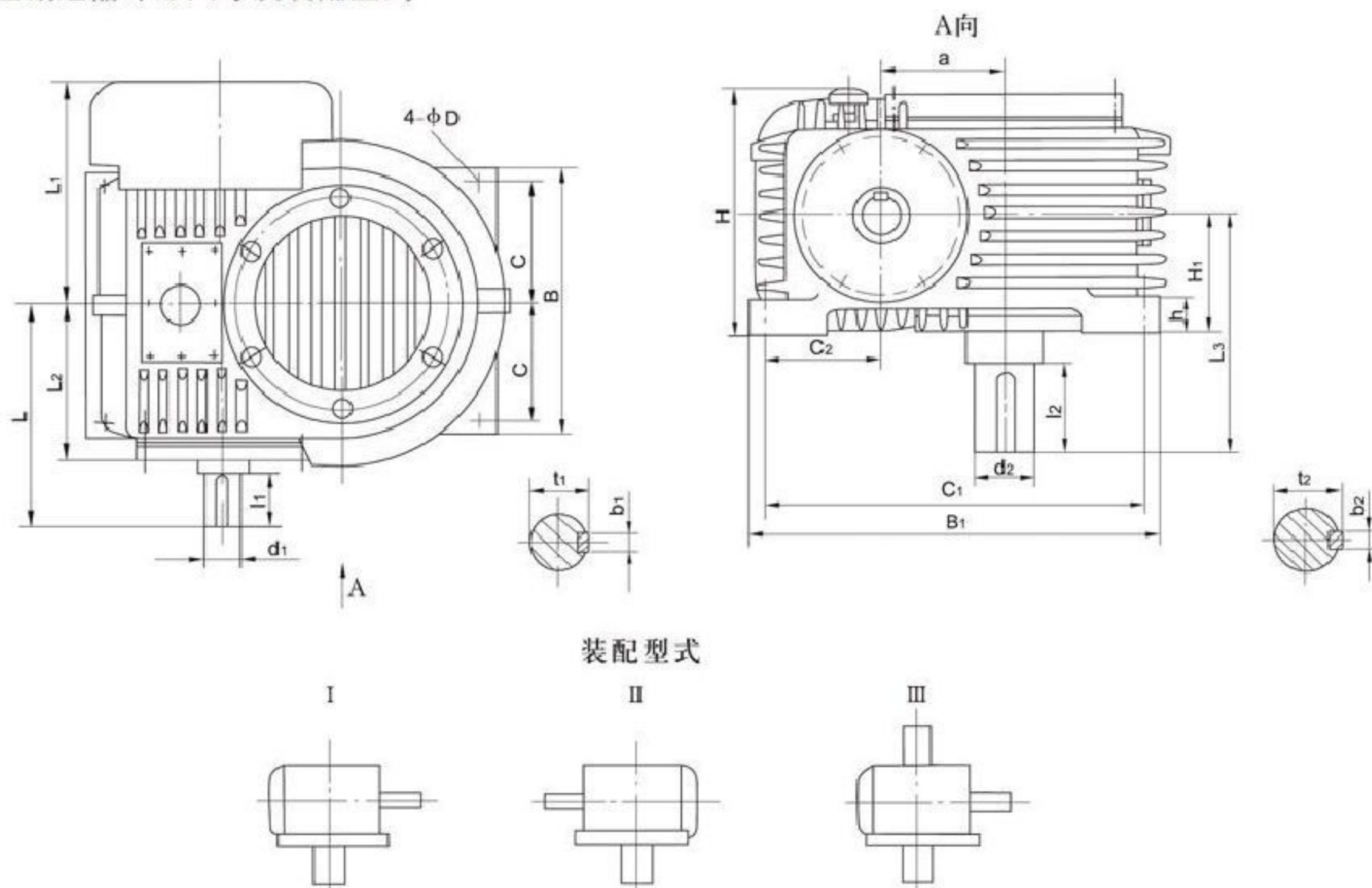
PWS 型减速器外形尺寸及装配型式
